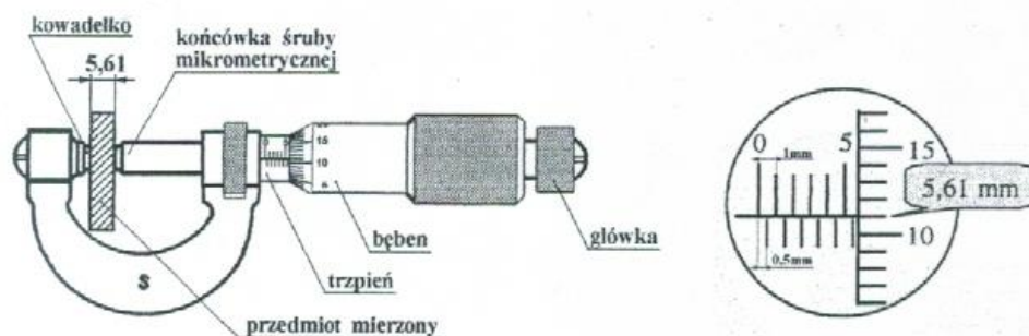
Rys. Śruba mikrometryczna.
